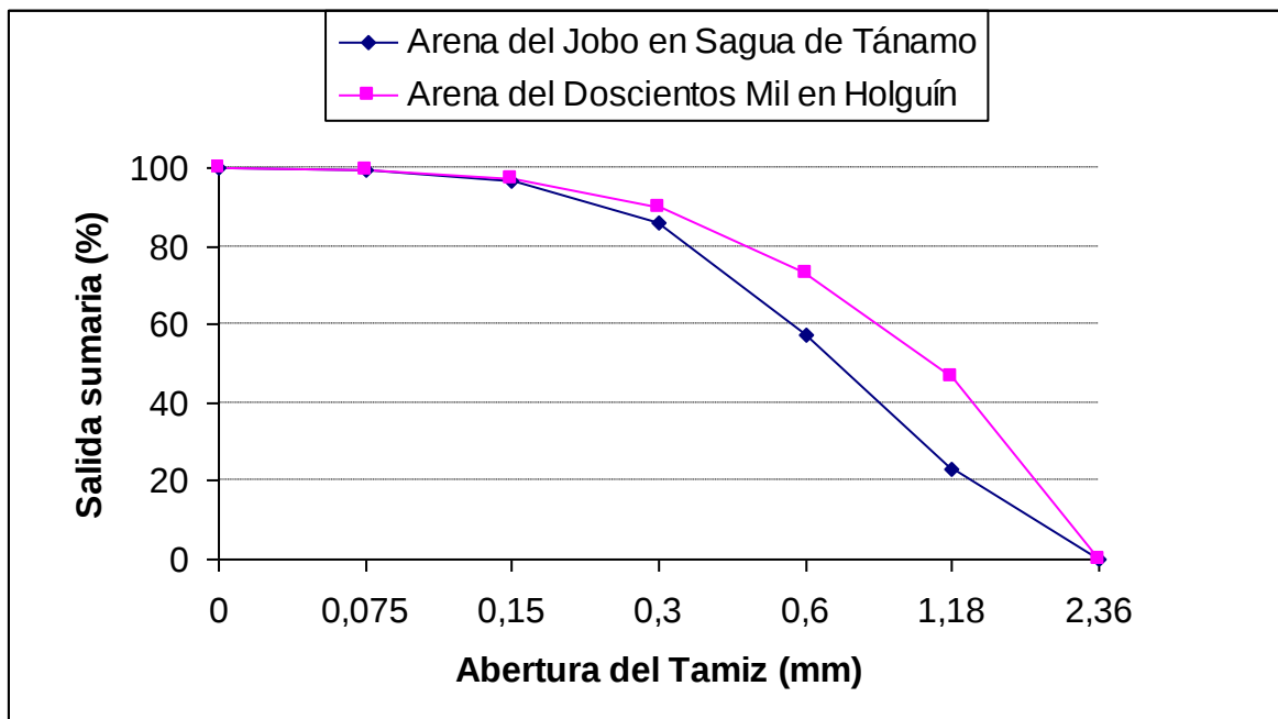
Figura 3.1. Característica de tamaño de la arena del Jobo en Sagua de Tánamo y Aguas Claras en Holguín
