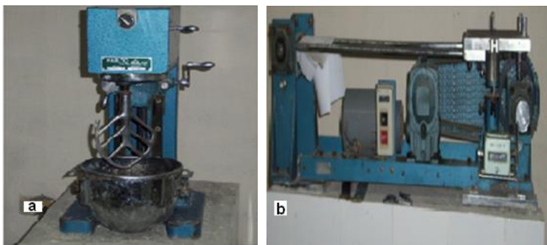
Figura 2.8. a) Mezcladora Maruto. b) Compactadora
