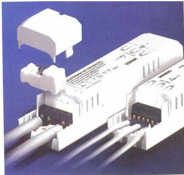
Figura 3. 2: Balasto para la familia TL – 80
