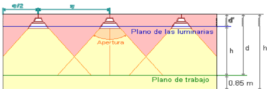
Figura 8: Apertura del haz de luz
