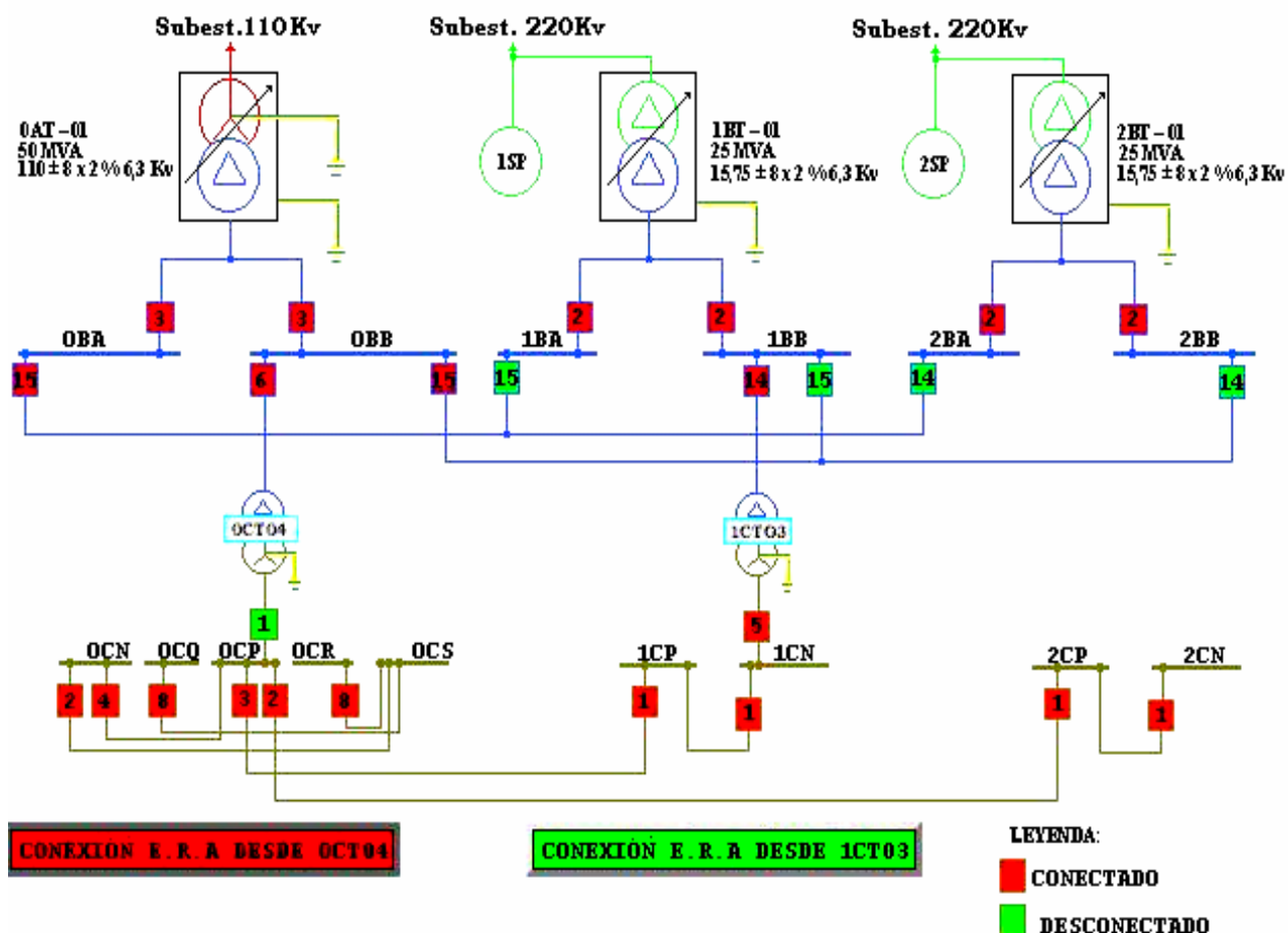
Figura #1: Esquema del sistema de alumbrado y climatización (variante # 1.)
