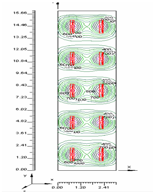
Figura 3. 6: Distribución de los lux que llegan Mando Eléctrico
