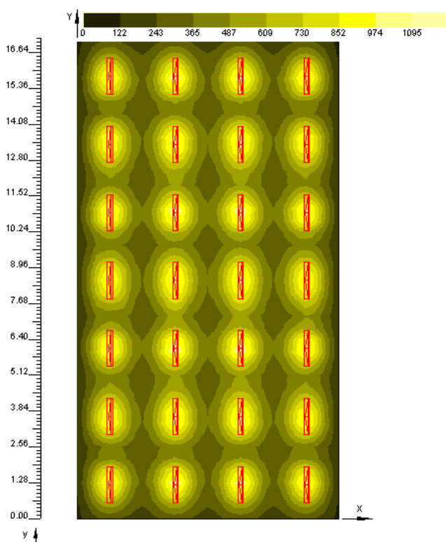
Figura 3. 4: Diagrama isolux
