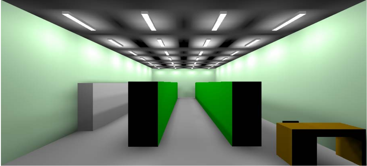
Figura 3. 5: Simulación con la propuesta realizada.
